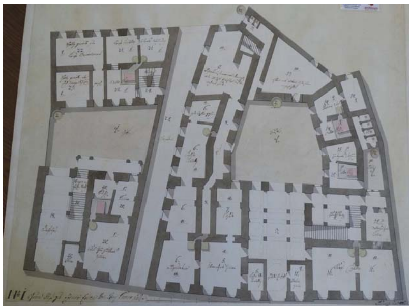
Obr. č. 1/ prízemie
