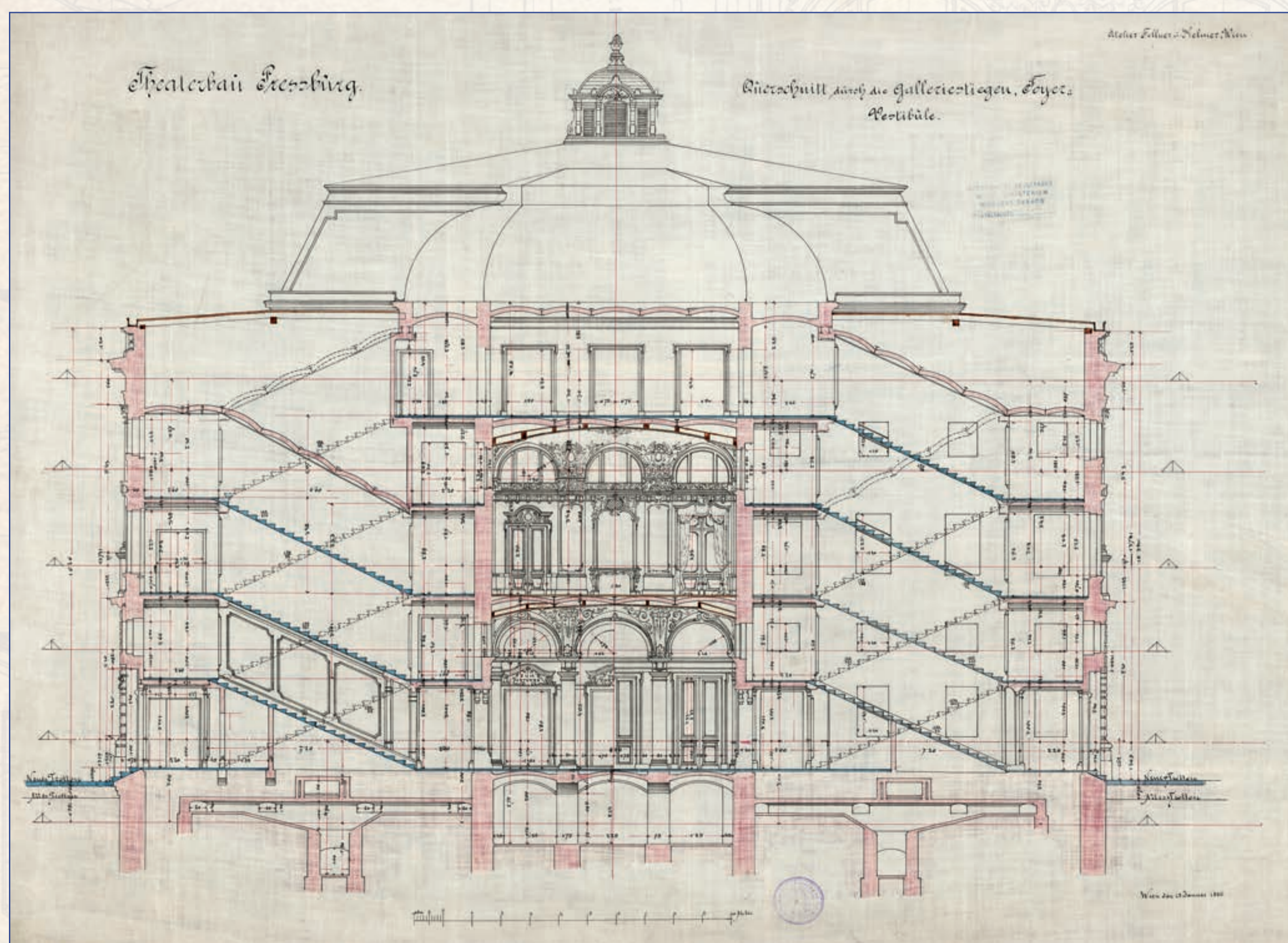
Projekt prestavby divadla architektov Ferdinanda Fellnera ml. a Hermanna Gottlieba Helmera
