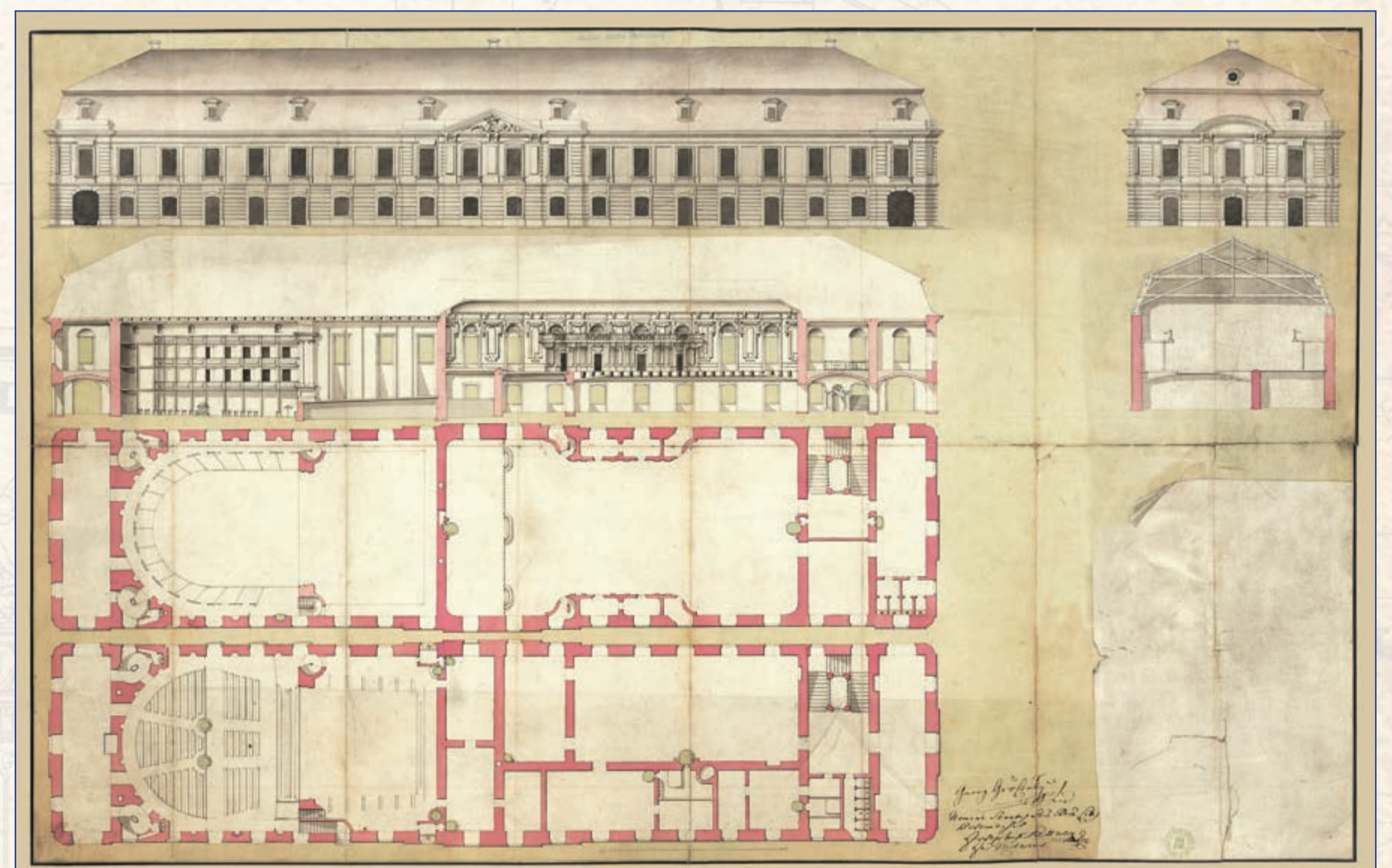
Plány Bratislavského mestského divadla – prvého kamenného divadla v Hornom Uhorsku
